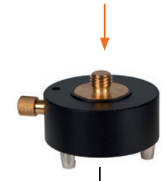
Bestell-Nr. 482 011 Drehbarer Dreifuß-Adapter mit 5/8" Gewinde zur Aufnahme von Prismensystemen mit 5/8". Steckzapfen mit Ø 34 mm Innengewinde. Farbe: schwarz
